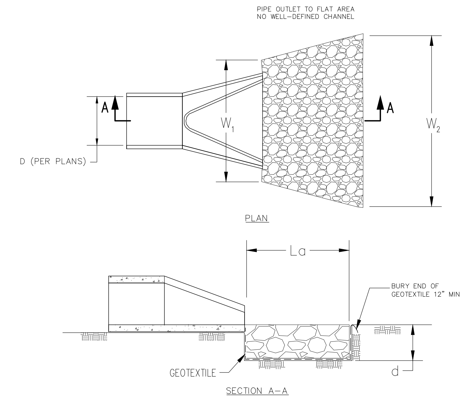
RIP RAP DETAIL OUTLET PROTECTION N.T.S.
