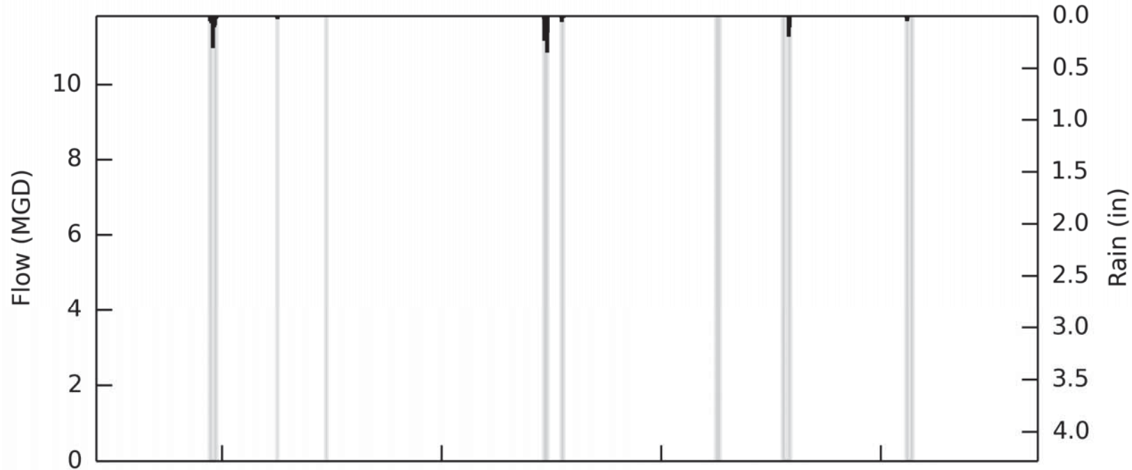
Meter CSO052B - 6/2016 RG: Anthony Basin: St Joe Conduit Diameter: 30
