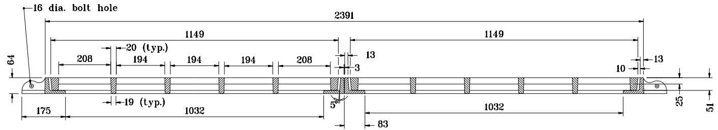
SECTION A-A
