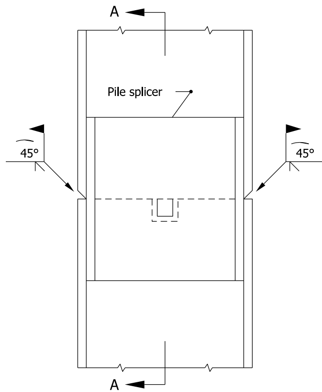
ELEVATION
