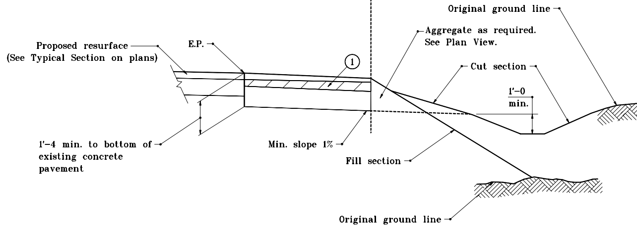
ELEVATION
