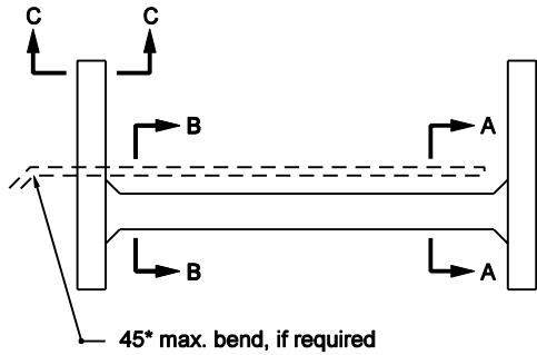
PLAN - END BENT
