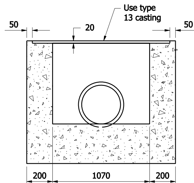
SECTION A-A INLET TYPE R (CONC.)
