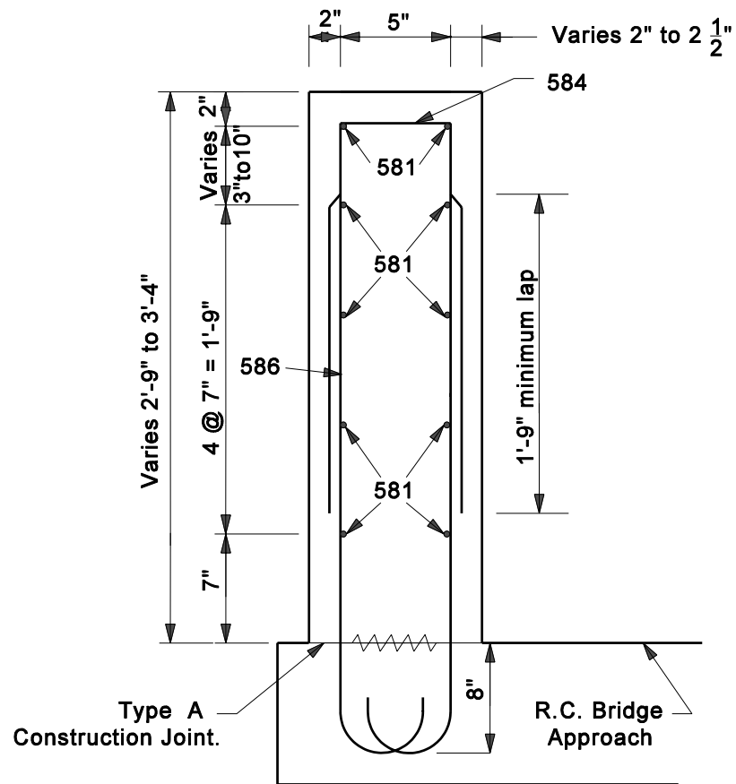
SECTION D-D
