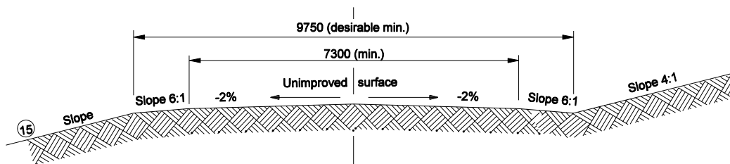
SECTION D-D
