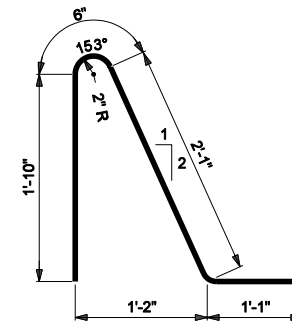
591a x 5'-6"
