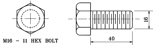
M16 - 11 HEX BOLT
