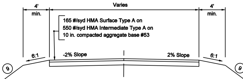
SECTION D-D
