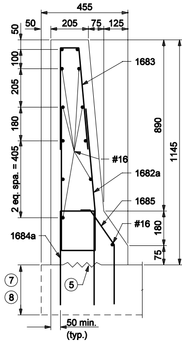
SECTION A-A
