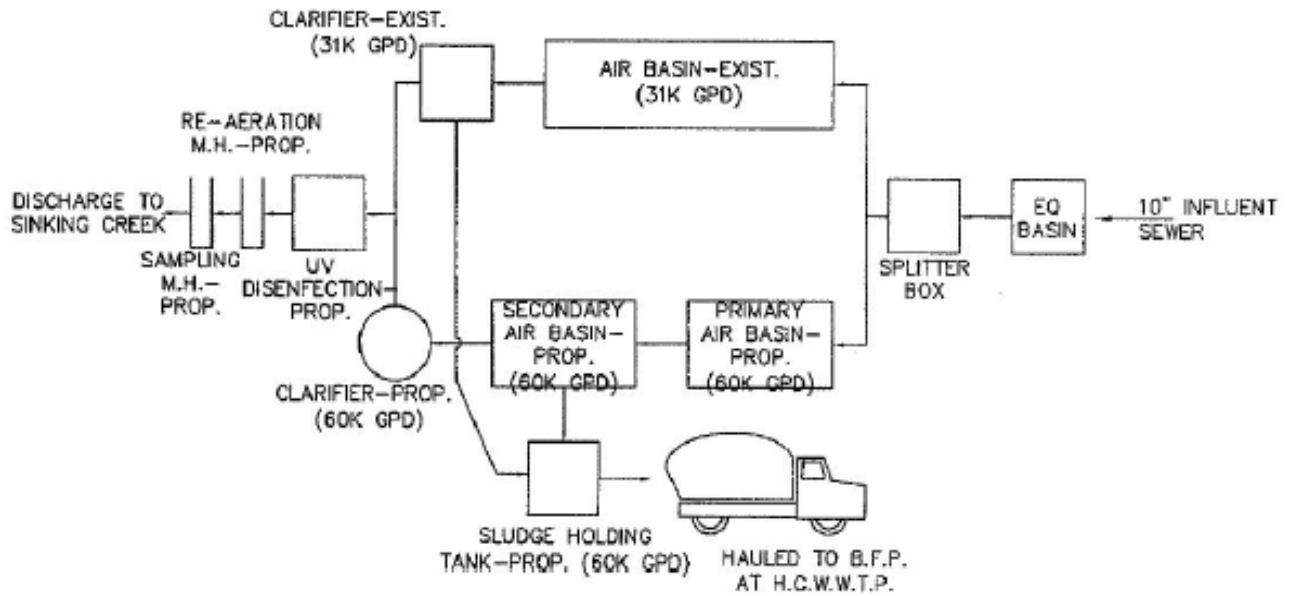
FLOW DIAGRAM N.T.S.
