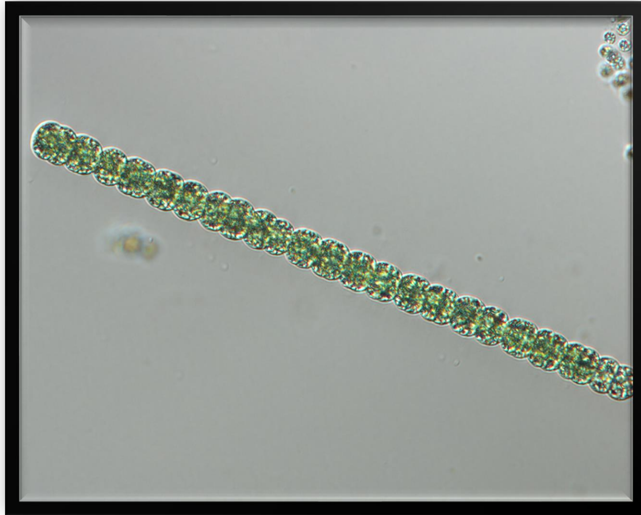
Anatoxin-a
