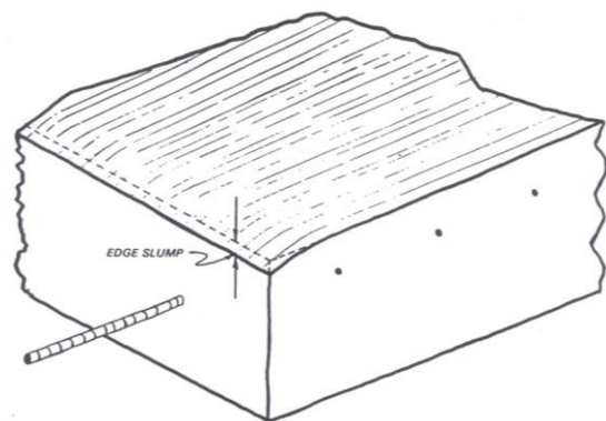
Figure 6-12 Edge Slump
